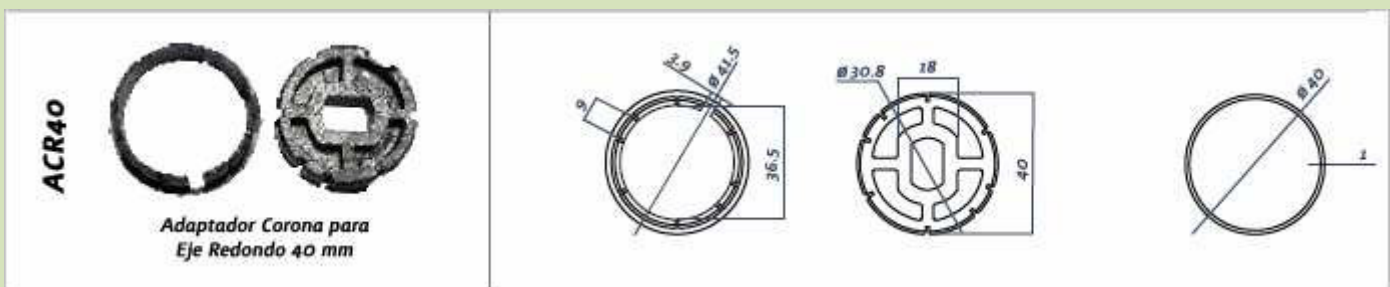
Referencia ACR40 Adaptador corona para eje redondo de 40 mm Ø Precio 5 € + iva
