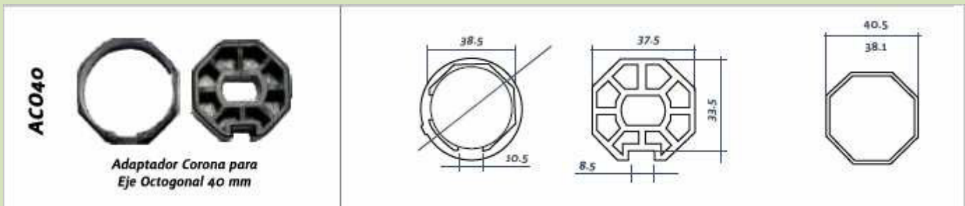
Referencia: ACO40 Adaptador corona para eje octagonal de 40 mm. Ø Precio 5€ + iva
